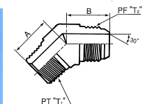
名称 オス45° エルボ 品名 1035
