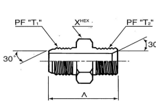
名称 オススイベルコネクター 品名 1018
