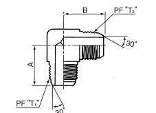
名称 オスオスフレア90° エルボ 品名 1020
