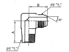
名称 オス90° エルボ 品名 1034
